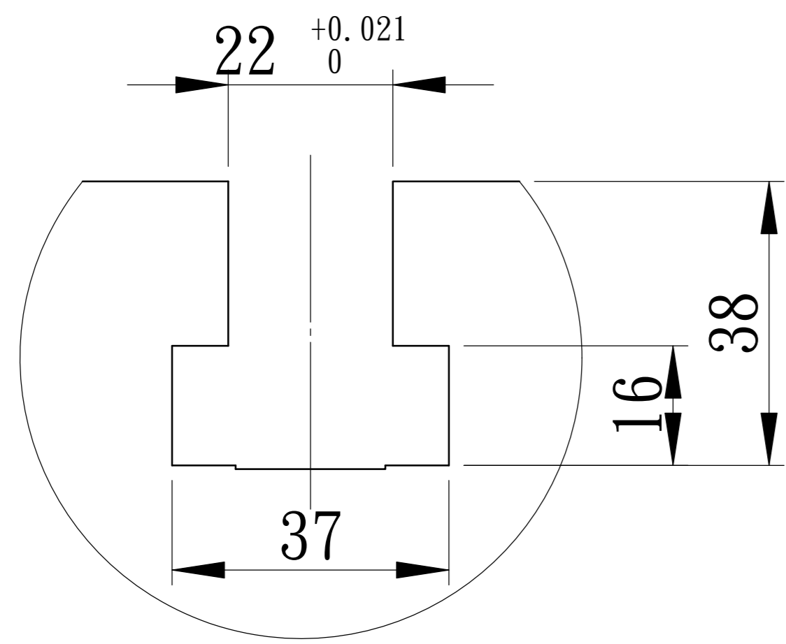
T槽詳圖 (1:2)
